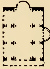
Fig. 112 — Planta della «basilica Nova» (basilica di Costantino) a Roma (a. 310-312)
